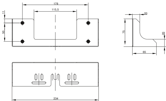
Рисунок 2 – Кронштейн / Figure 2. Bracket
