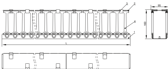
Рисунок 1 – Кабель-органайзер (1 – основание, 2 – крышка, 3 – скрепка, 4 – стойка) / Figure 1. Cable organizer (1 – base, 2 – cover, 3 – clip, 4 – rack)
