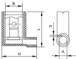
Рисунок 9 – Разъём РпФим
