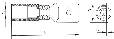
Рисунок 10 – Разъём РпИп-т
