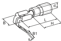
Рисунок 2 – Разъём РпИю
