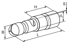
Рисунок 4 – Разъём РшИп
