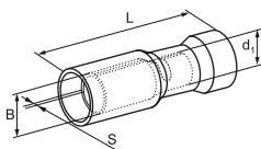
Рисунок 5 – Разъём РшИм
