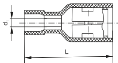
Рисунок 7 – Разъём РпИм-н
