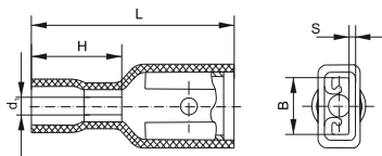
Рисунок 6 – Разъём РпИмп
