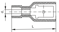
Рисунок 8 – Разъём РпИп-н
