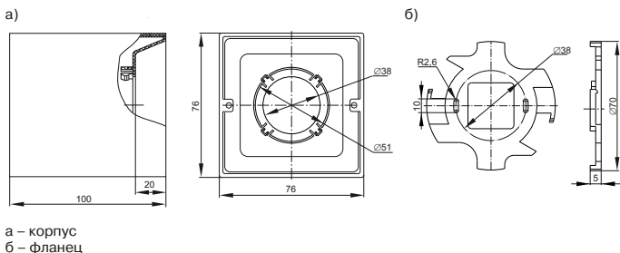
Рисунок 7 – Светильник 4112
