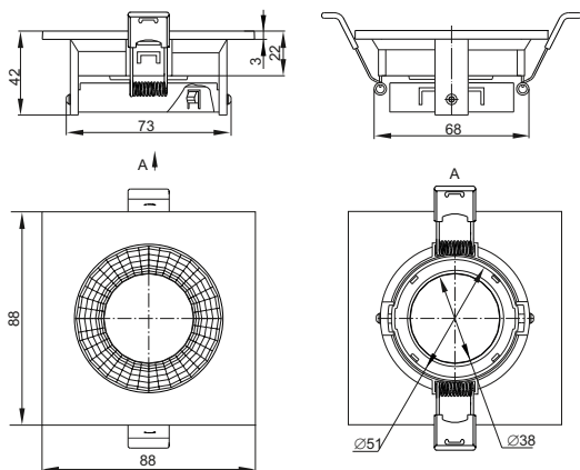
Рисунок 5 – Светильник 4110
