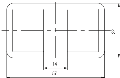
Рисунок 3 – Колпачок защитный IP65 AD22-D1 для прямоугольной двояной кнопки
