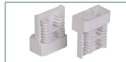
Держатели DIN-рейки ступенчатого типа
