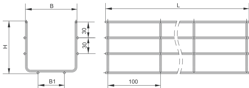
Рисунок / Figure / Сурет 3 – Лоток проволочный высотой H = 100 мм / Wire mesh cable tray with a height H = 100 mm / Биіктігі H = 100 мм сымды науа
