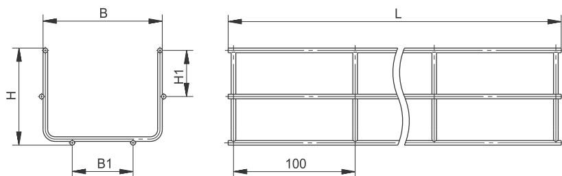
Рисунок / Figure / Сурет 2 – Лоток проволочный высотой H = 80 мм / Wire mesh cable tray with a height H = 80 mm / Биіктігі H = 80 мм сымды науа
