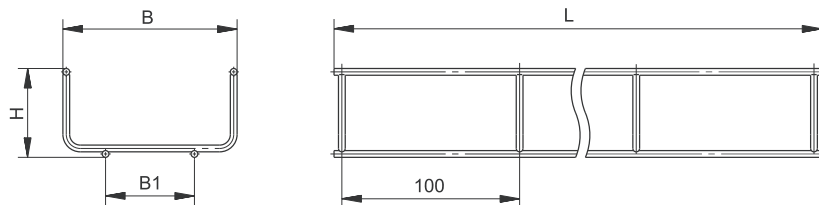
Рисунок / Figure / Сурет 1 – Лоток проволочный высотой H = 35, 50 мм / Wire mesh cable tray with a height H = 35, 50 mm / Биіктігі H = 35, 50 мм сымды науа
