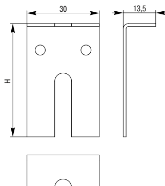
Рисунок 4 – Держатель крышки лотка боковой / Figure 4 – Side tray cover holder
