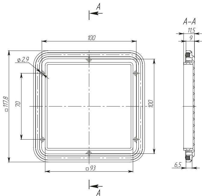
Рисунок / Figure / Сурет 1— Окошко смотровое для корпусов полиэфирных / Sight window for polyester enclosures / Полиэстерлі корпустарға арналған бақылау тексеру терезесі
