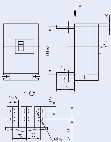
Рисунок 3 – Выключатели типов ВА52-41, ВА53-41, ВА55-41, ВА56-41 стационарного исполнения с ручным приводом для заднего присоединения шиной
