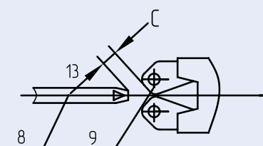
Врубные контакты выключателя в положении расчленения (разъединителя)
