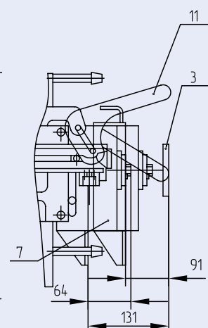
Рисунок 7 – Выключатели типов ВА52-41, ВА53-41, ВА55-41, ВА56-41 в выдвижном исполнении на номинальный ток 1000 А
