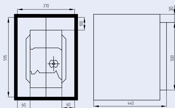
Рисунок 11 – Минимальные размеры ячейки, в которой может быть установлен выключатель выдвжного исполнения на номинальные токи 250, 400, 630 А
