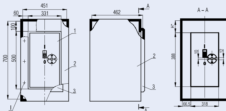
Рисунок 10 – Минимальные размеры ячейки, в которой может быть установлен выключатель выдвжного исполнения на номинальный ток 1000 А
