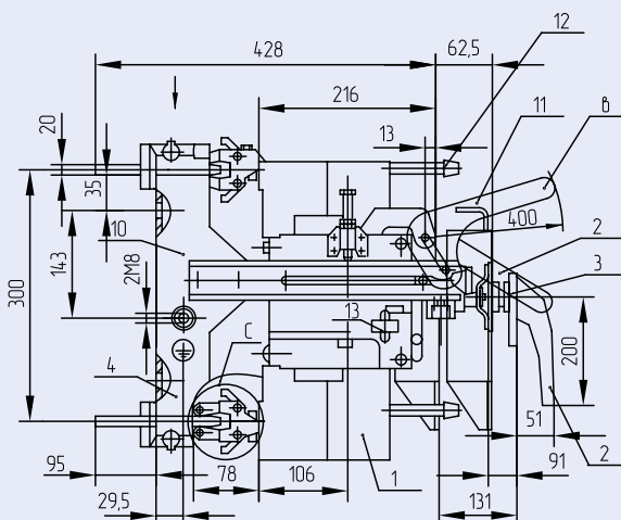
Рисунок 7 – Выключатели типов ВА52-41, ВА53-41, ВА55-41, ВА56-41 в выдвижном исполнении на номинальный ток 1000 А
