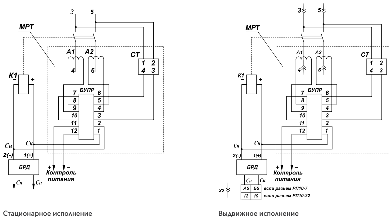
Рисунок 22 – Схема электрическая принципиальная выключателей постоянного тока
