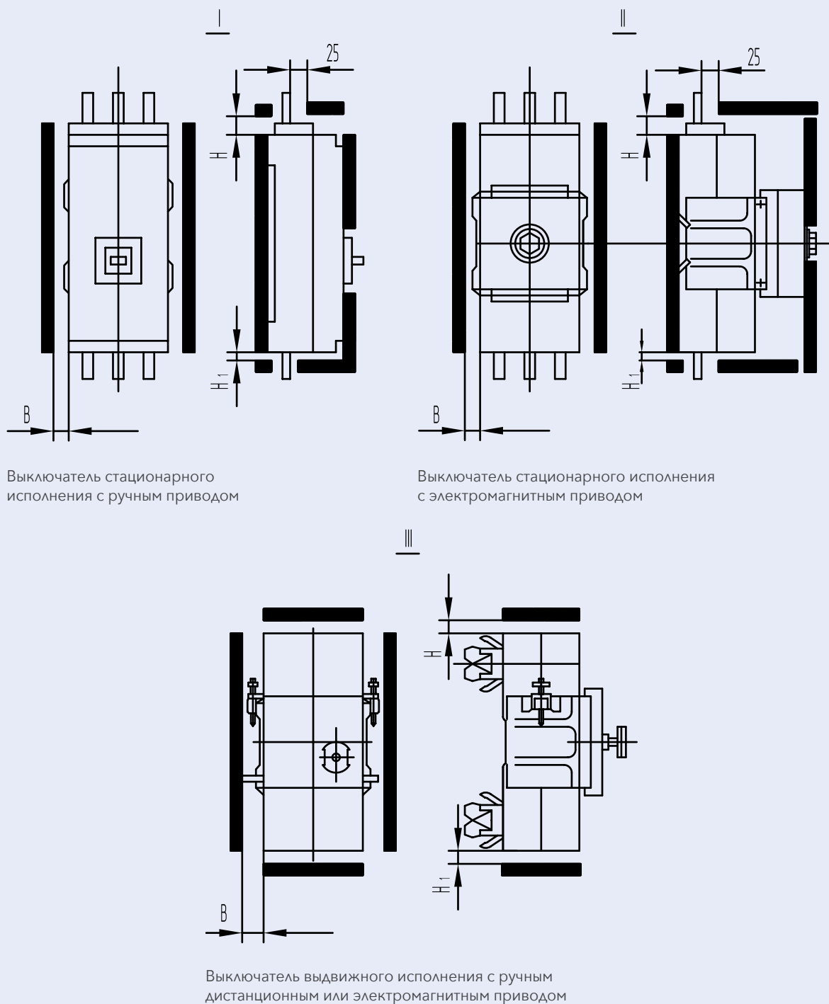
Рисунок 9 – Расположение выключателей серии ВА50-41 в распределительном устройстве
