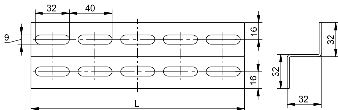
Рисунок 10 – Профиль перфорированный Z-образный K241
