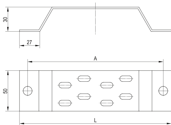
Рисунок 6 – Стойка настенная
