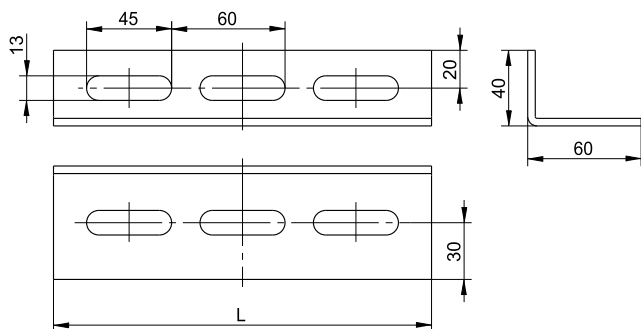
Рисунок 13 – Профиль перфорированный L-образный ГЭМ K242
