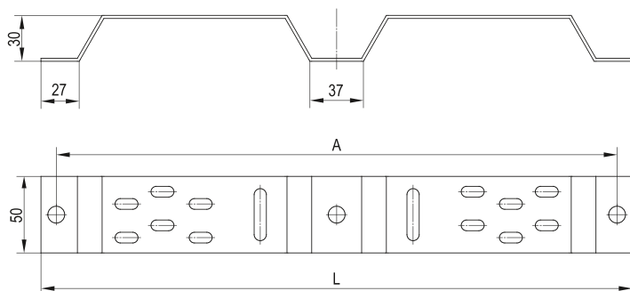
Рисунок 7 – Стойка настенная
