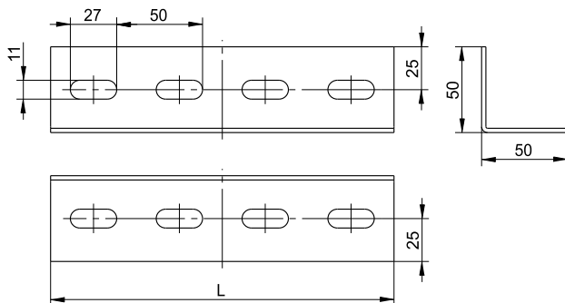
Рисунок 14 – Профиль перфорированный L-образный L-2,5
