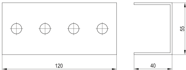
Рисунок 3 – Профиль настенный
