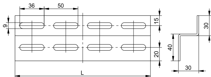
Рисунок 8 – Профиль перфорированный Z-образный K238
