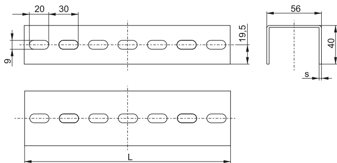
Рисунок 15 – Профиль перфорированный П-образный
