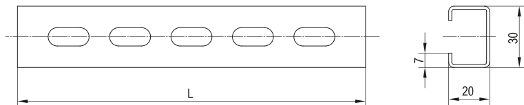
Рисунок 1 – Профиль перфорированный С-образный
