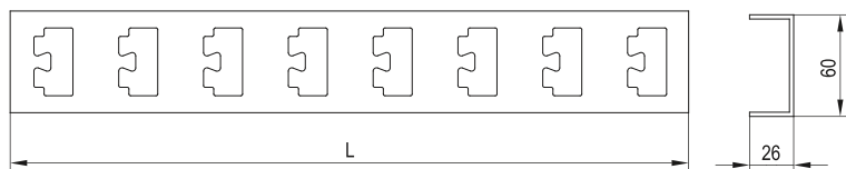
Рисунок 5 – Стойка кабельная
