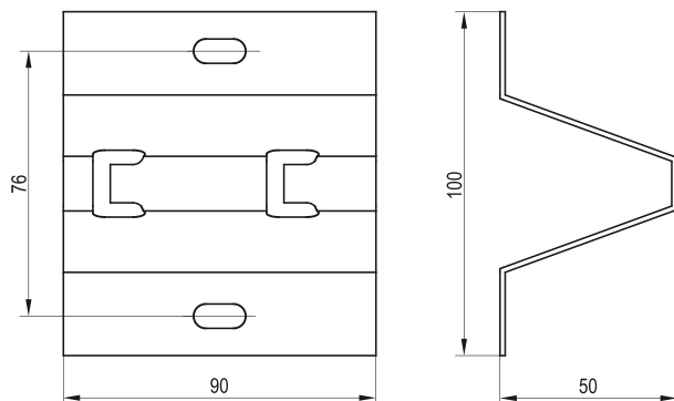
Рисунок 4 – Стойка напольная 100
