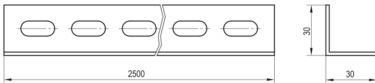
Рисунок 2 – Профиль перфорированный L-образный
