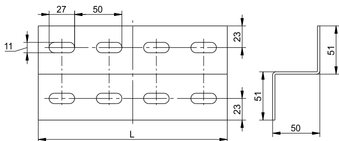
Рисунок 11 – Профиль перфорированный Z-образный L-2,5
