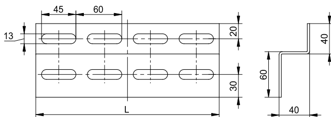
Рисунок 9 – Профиль перфорированный Z-образный K239
