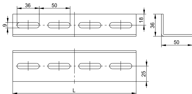
Рисунок 12 – Профиль перфорированный L-образный ГЭМ К237
