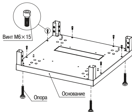
Рисунок 1 – Нижнее основание
