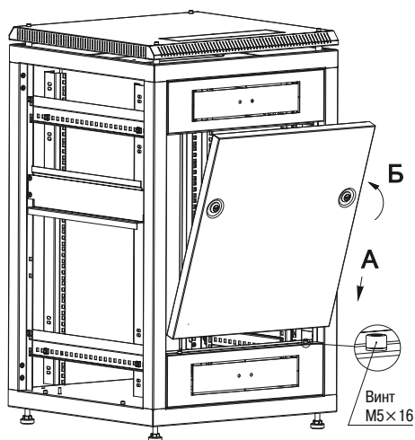
Рисунок 9 – Установка панели задней в шкаф
