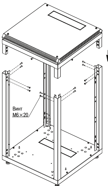
Рисунок 4 – Установка «основания-крыши»
