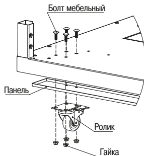
Рисунок 17 – Установка роликов
