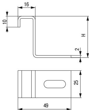
Рисунок 9 – Скоба для крепления лотка
