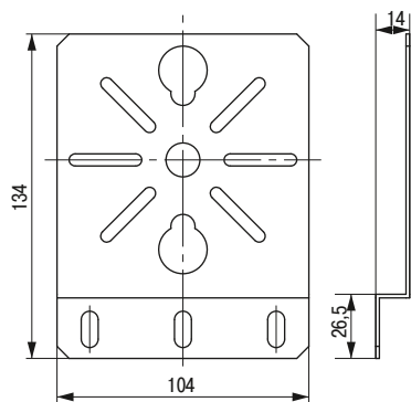
Рисунок 2 – Пластина монтажная вертикальная
