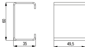
Рисунок 13 – Распорка для П-образного профиля
