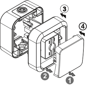
Рисунок 1 – Порядок монтажа выключателя / Figure 1 – Switch installation procedure / 1 сурет – Ажыратқышты монтаждау тәртібі
