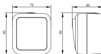
Рисунок 4 – Основные габаритные размеры / Figure 1 – Main overall dimensions / 4 сурет – Негізгі габариттік өлшемдері
