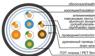
Рисунок 3 – Конструкция кабеля типа F/UTP (количество жил 2×2) / Figure 3 – Cable design of F/UTP type (amount of cores 2×2)
