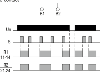
Рисунок 6 – Функциональная диаграмма реле ORM двухконтактные. Режим управления 2 / Figure 6 - Functional diagram of the ORM two-contact relays. Operation mode 2
