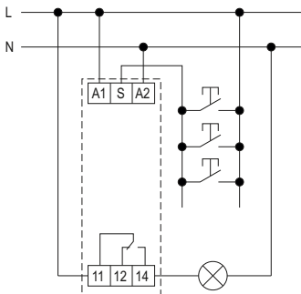
ORM одноконтактные / single-contact
