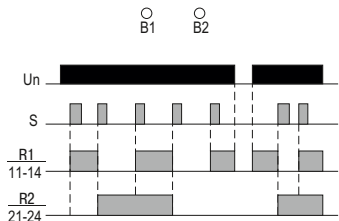
Рисунок 5 – Функциональная диаграмма реле ORM двухконтактные. Режим управления 1 / Figure 5 - Functional diagram of the ORM two-contact relays. Operation mode 1
