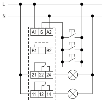
ORM 2 двухконтактные / double-contact
