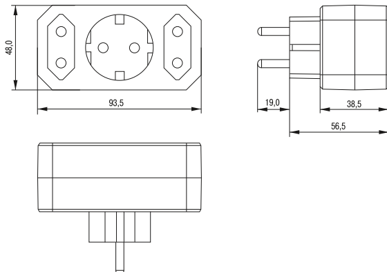
Рисунок 1 – Тройник Т-01/01-2
