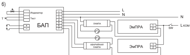
а) Схема подключения с ЭмПРА для однолампового светильника.
