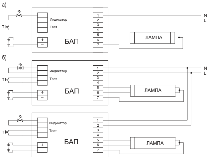
а) Схема подключения без пускорегулирующего аппарата для однолампового светильника.
