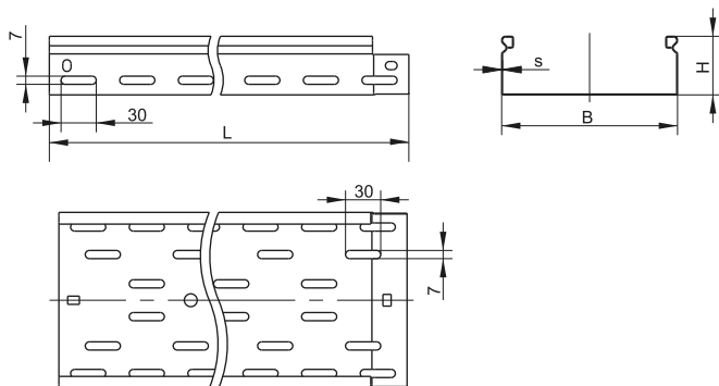
Рисунок 1. Габаритные размеры лотка перфорированного серии ESCA
