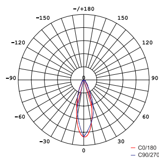
КСС К (30°)
