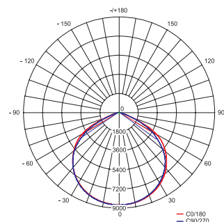
Тип Д (120°)
