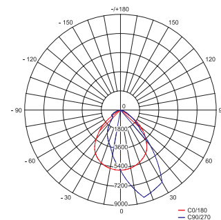
Тип «Кососвет»
