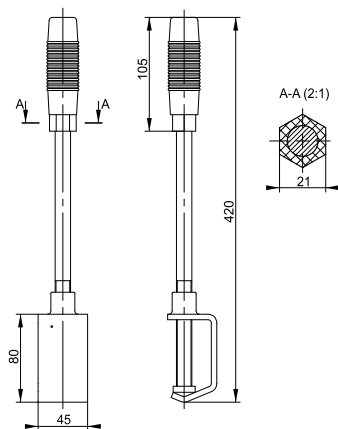
Рисунок 1 – Габаритные размеры струбицы
