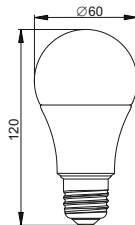
Рисунок 3 – Лампа LED ALFA A60 20 Вт цоколь E27
