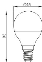
Рисунок 8 – Лампа LED ALFA G45 10 Вт цоколь E14
