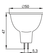
Рисунок 13 – Лампа LED ALFA MR16 6 Вт, 8 Вт цоколь GU5,3
