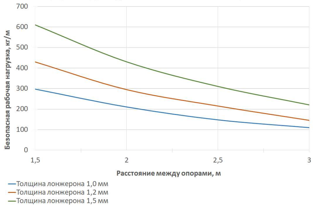
График нагрузок для лотков LESTA с высотой борта 100 мм
