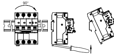
Демонтаж АВДТ34 на DIN-рейку / Dismantling of AVDT34
