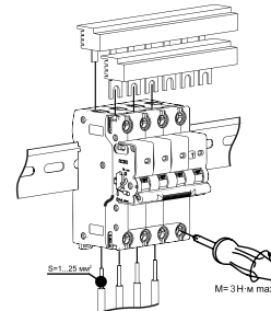
Пример монтажа АВДТ34 / Example of AVDT34 mounting
