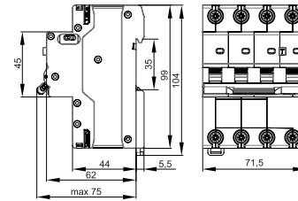
Габаритные и установочные размеры АВДТ34 / Overall and mounting dimensions of AVDT34
