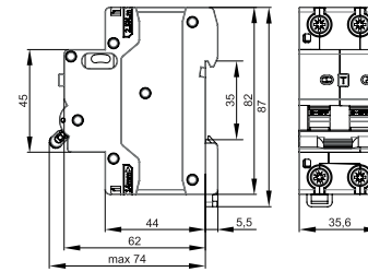
Габаритные и установочные размеры АВДТ32 / Overall and mounting dimensions of AVDT32
