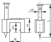
Скоба плоская
