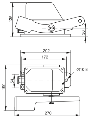
Рисунок 2. Габаритные и установочные размеры выключателей КУ-703 У1
