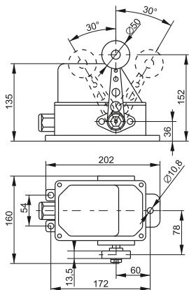
Рисунок 1. Габаритные и установочные размеры выключателей КУ-701 У1
