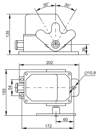
Рисунок 3. Габаритные и установочные размеры выключателей КУ-704 У1
