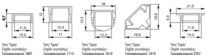
Рисунок 1 – Габаритные размеры профиля/ Figure 1 – Overall dimensions of the profile/ 1-sýret – Profildiriň gabarittik ölçemleri/ Рисунок 1 – Габаритні розміри профілю
