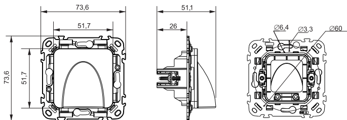
Рисунок 2 – Габаритные и установочные размеры вывода кабеля / Figure 2 – Overall and installation dimensions of the cable outlet / 2-сурет – Кабельді шығарудың габаритті және орнату өлшемдері
