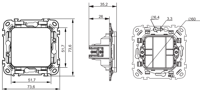
Рисунок 1 – Габаритные и установочные размеры заглушки / Figure 1 – Overall and installation dimensions of the plug / 1-сурет – Бітеуіштің габаритті және орнату өлшемдері
