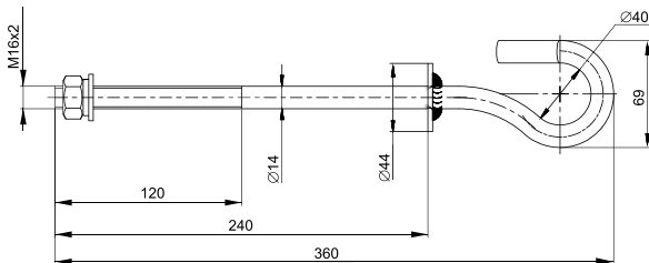
а) крюк монтажный / mounting hook / монтаждау ілмері В 16/240
