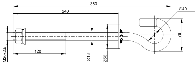
б) крюк монтажный / mounting hook / монтаждау ілмері В 20/240
