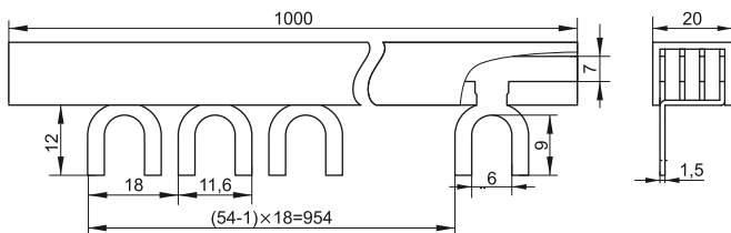
Рисунок 8 – Шина типа FORK 4P 63 А шаг 18 мм
