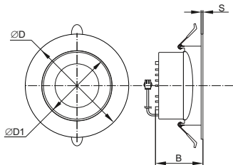
Рисунок 1 – Габаритные размеры ДВО 1811 PRO – ДВО 1813 PRO
