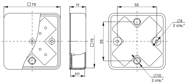
Рисунок / Figure / Сурет 2 – Коробки / Boxes / Қораптары UKO10-075-075...
