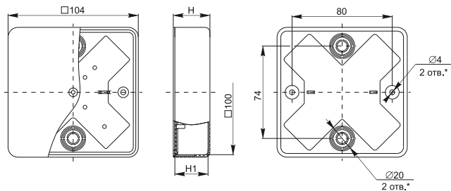
Рисунок / Figure / Сурет 3 – Коробки / Boxes / Қораптары UKO10-100-100...
