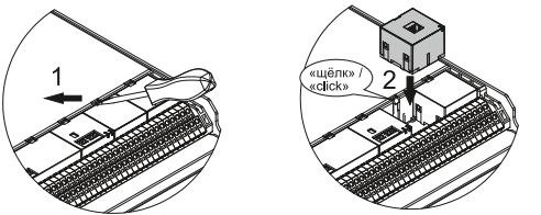
Рисунок 2 – Установка модуля передачи данных / Figure 2 – Installation of the communication module
