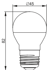
Рисунок 16 – Лампа LED Globe G45, 7 Вт, цоколь E27 / Figure 16 – LED-G45 lamp, 7 W, E27 lamp base
