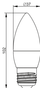
Рисунок 12 – Лампа LED Candle C37, 7 Вт, цоколь E27 / Figure 12 – LED-C37 lamp, 7 W, E27 lamp base
