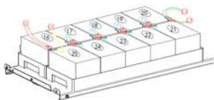
Рисунок 40 – Схема соединения батарей четвёртого яруса
