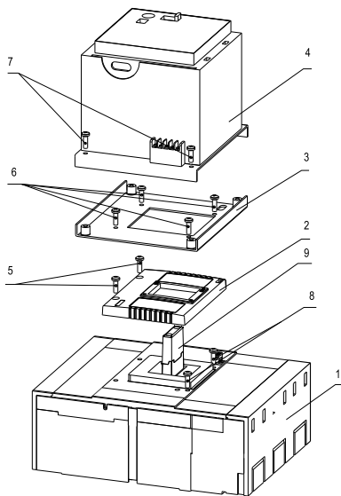
Рисунок 3 – Монтаж электропривода
