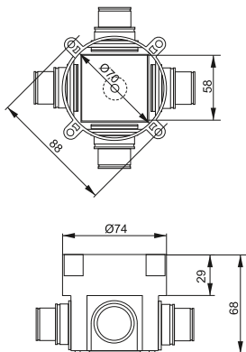
Рисунок 2 – Габаритные размеры коробки установочной d=70×72 мм для монолитного строительства, черная
