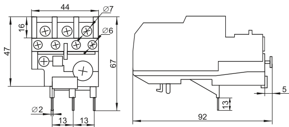
Рисунок 2. Габаритные и установочные размеры реле РТИ-1301... РТИ-1322.
