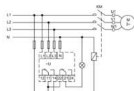
b) ORF-SN-070-400VAC С функцией контроля нейтральной линии
