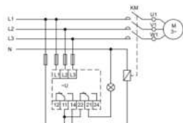
a) ORF-SP-130-850VAC Без функции контроля нейтральной линии
