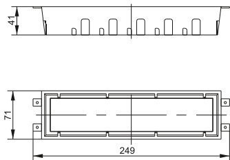
Рисунок 3 – Коробка приборная ONFLOOR / Figure 3 – Instrument box ONFLOOR / 3-suret – ONFLOOR aspartuq qoraby / Рисунок 3 – Коробка приладова ONFLOOR
