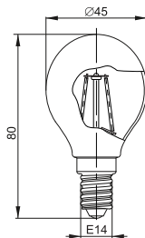
Рисунок 4 – Лампа LED-G45 серия 360° 5 Вт, 7 Вт цоколь E14
