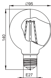
Рисунок 10 – Лампа LED-G95 серия 360° 6 Вт, 8 Вт цоколь E27
