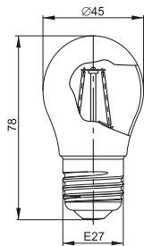
Рисунок 5 – Лампа LED-G45 серия 360° 5 Вт, 7 Вт цоколь E27
