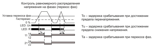
Рисунок 4 – Функциональные диаграммы реле ORF-06D; ORF-08D
