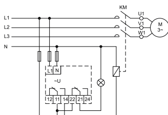
г) ORF-06D; ORF-08D с функцией контроля нейтральной линии
