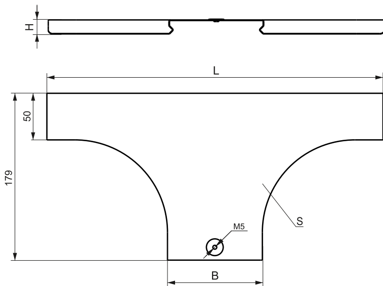
Рисунок 1 – Крышка отвода Т-образного плавного серии ESCA
