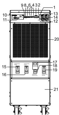
Рисунок 6 – Элементы задней панели ИБП серии ELECTRA OB 100 – 160 кВА
