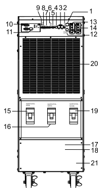
Рисунок 7 – Элементы задней панели ИБП серии ELECTRA OB 180 – 200 кВА
