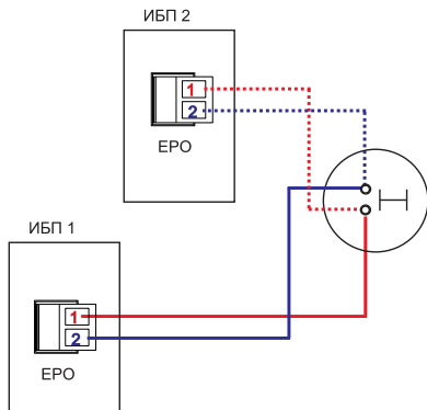
Рисунок 27 –Схема подключения контактов ЕРО между ИБП
