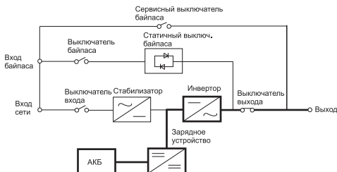
Рисунок 9 – Схема работы ИБП в режиме АКБ
