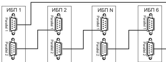
Рисунок 17 – Схема параллельного подключения
