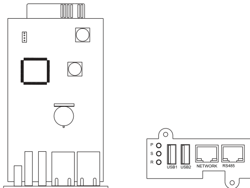
Рисунок 29 – Карта SNMP
