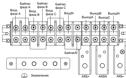
Рисунок 13 – Обозначение клемм питания ИБП серии ELECTRА OB 80 кВА
