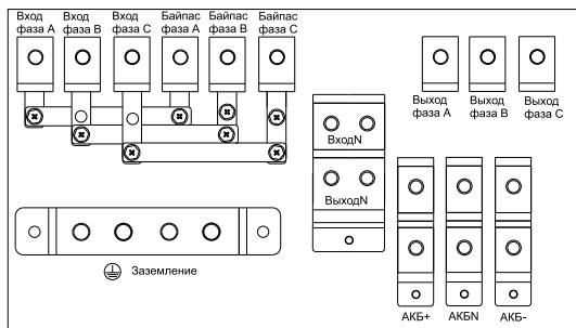
Рисунок 14 – Обозначение клемм питания ИБП серии ELECTRА OB 100 –160 кВА
