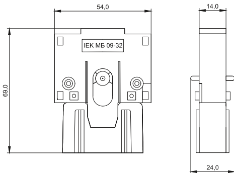
а) Механизм блокировки для КМИ (09А-32А) / a) Locking mechanism for KMI (09А-32А)
