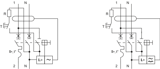
a) АВДТ типа AC / RCBO of AC type
