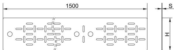
Рисунок 19 – Вставка донная для лотка LESTA 1500 / Figure 19 – Bottom ferrule for LESTA tray 1500 / 19-keste – LESTA 1500 nauağa arналğan tüptik endirmesi / Рисунок 19 – Вставка донна для лотка LESTA 1500
