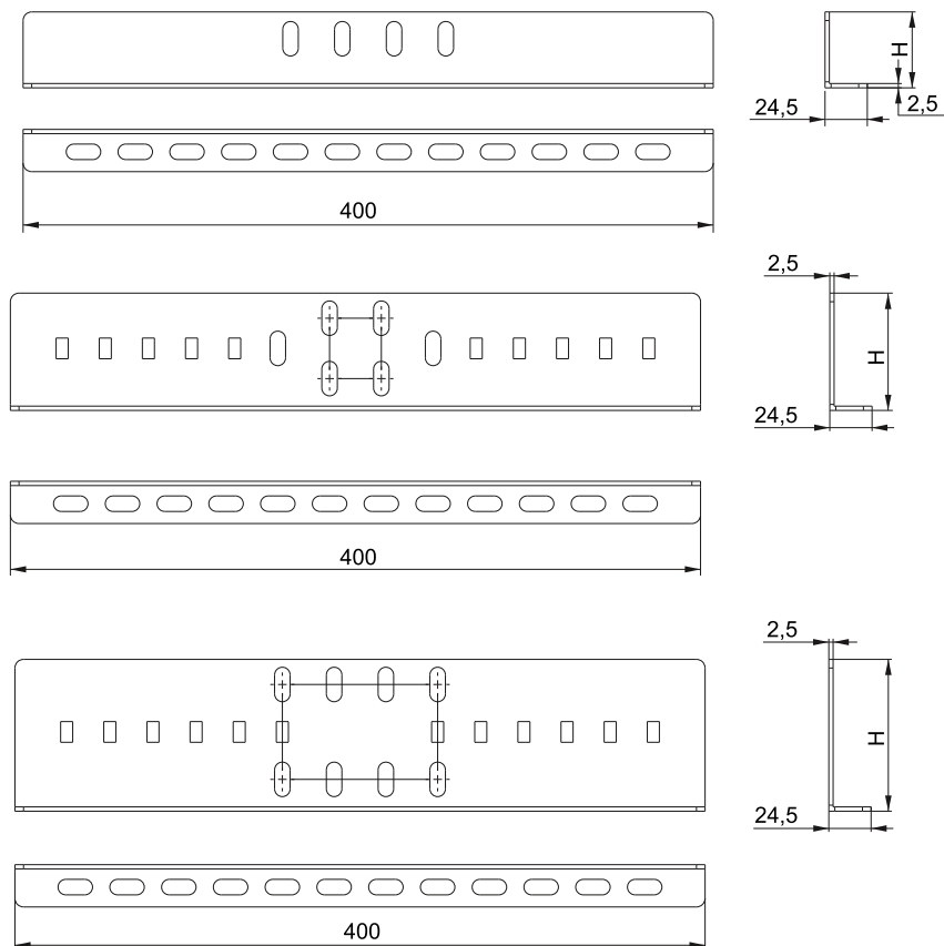
Рисунок 18 – Пластина соединительная усиленная LESTA / Figure 18 – LESTA armored coupler / 18-keste – LESTA küşeytilgen bailyanystyryuş plastinasy / Рисунок 18 – Пластина з'єднувальна посилена LESTA
