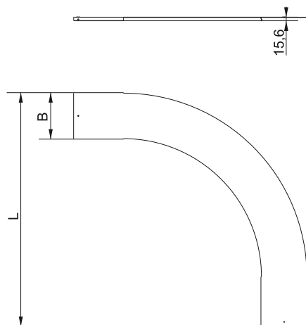
Рисунок 8 – Крышка поворота лестничного LESTA на 90 гр. R600 / Figure 8 – LESTA ladder cover 90 deg. turn R600 / 8-suret – LESTA satyly бүрлмасынүң қақағау 90 гр. R600 / Рисунок 8 – Крышка повороту драбинного LESTA на 90 гр. R600
