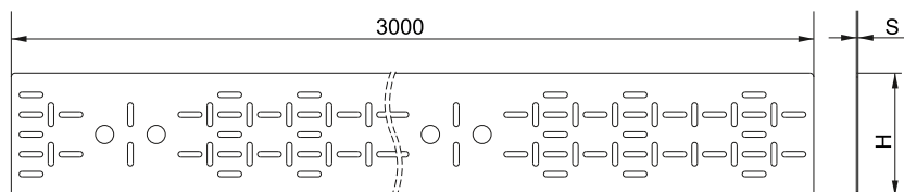
Рисунок 20 – Вставка донная для лотка LESTA 3000 / Figure 20 – Bottom ferrule for LESTA tray 3000 / 20-keste – LESTA 3000 nauağa arналğan tüptik endirmesi / Рисунок 20 – Вставка донна для лотка LESTA 3000
