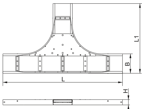
Рисунок 9 – Разветвитель лестничный Т-образный LESTA на 90 градусов R300 / Figure 9 – 90 degree LESTA T-shape ladder bracing device R300 / 9-suret – LESTA T-tärizdi satylyq tarmaқтағышт 90 gradys R300 / Рисунок 9 – Розгалужувач драбинний Т-подібний LESTA на 90 градусів R300
