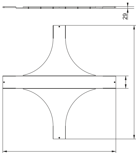
Рисунок 16 – Крышка крестовины лестничной LESTA R600 / Figure 16 – LESTA ladder cross-piece cover R600 / 16-suret – LESTA satylyq aigastyrmasynyn qaqpағу R600 / Рисунок 16 – Кришка хрестовини драбинної LESTA R600
