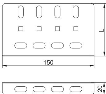
Рисунок 17 – Пластина соединительная LESTA / Figure 17 – LESTA coupler / 17-keste – LESTA bailanystyrғыs plastinasы / Рисунок 17 – Пластина з'єднувальна LESTA
