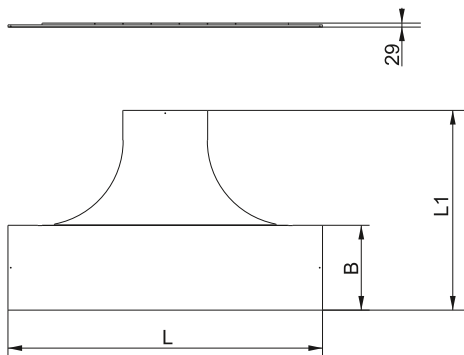
Рисунок 12 – Крышка разветвителя лестничного Т-образного LESTA на 90 градусов R600 / Figure 12 – 90 degree LESTA T-shape bracing device cover R600 / 12-suret – LESTA T-tärizdi satylyq tarmaqtağyştyn qaqpağ 90 gradyc R600 / Рисунок 12 – Крышка розгалужувача драбинного Т-подібного LESTA на 90 градусів R600
