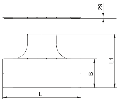
Рисунок 10 – Крышка разветвителя лестничного Т-образного LESTA на 90 градусов R300 / Figure 10 – 90 degree LESTA T-shape bracing device cover R300 / 10-suret – LESTA T-tärizdi satylyq tarmaқтағыштүң қақағау 90 gradys R300 / Рисунок 10 – Крышка розгалужувача драбинного Т-подібного LESTA на 90 градусів R300
