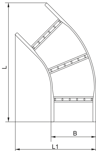
Рисунок 1 – Поворот лестничный LESTA на 45 гр. R300 / Figure 1 – LESTA ladder 45 deg. turn R300 / 1-suret - LESTA satyly bürilmasy 45 gr. R300 / Рисунок 1 – Поворот драбинный LESTA на 45 гр. R300
