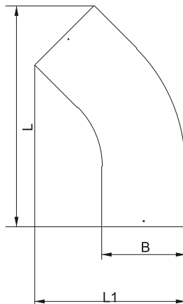
Рисунок 2 – Крышка поворота лестничного LESTA на 45 гр. R300 / Figure 2 – LESTA ladder cover 45 deg. turn R300 / 2-suret – LESTA satyly bürilmasyñyñ qaqraǵy 45 gr. R300 / Рисунок 2 – Крышка повороту драбинного LESTA на 45 гр. R300
