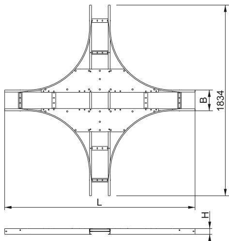
Рисунок 15 – Крестовина лестничная LESTA R600 / Figure 15 – LESTA ladder cross-piece R600 / 15-suret – LESTA satylyq aigastyrması R600 / Рисунок 15 – Хрестовина драбинна LESTA R600
