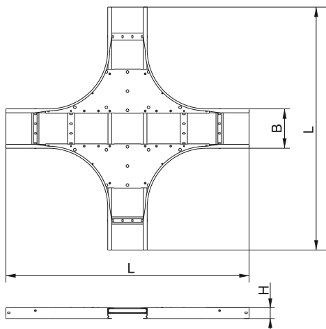
Рисунок 13 – Хрестовина лестничная LESTA R300 / Figure 13 – LESTA ladder cross-piece R300 / 13-suret – LESTA satylyq aqastymasy R300 / Рисунок 13 – Хрестовина драбинна LESTA R300
