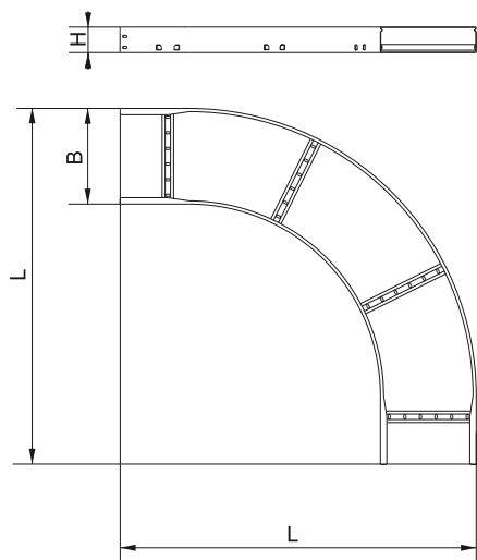
Рисунок 7 – Поворот лестничный LESTA на 90 гр. R600 / Figure 7 – LESTA ladder 90 deg. turn R600 / 7-suret – LESTA satyly бүрлмасы 90 гр. R600 / Рисунок 7 – Поворот драбинний LESTA на 90 гр. R600
