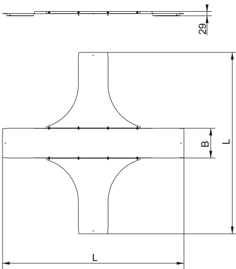
Рисунок 14 – Крышка хрестовины лестничной LESTA R300 / Figure 14 – LESTA ladder cross-piece cover R300 / 14-suret – LESTA satylyq aqastymasynyn qaqpağy R300 / Рисунок 14 – Крышка хрестовины драбинної LESTA R300
