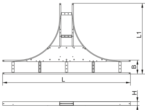
Рисунок 11 – Разветвитель лестничный Т-образный LESTA на 90 градусов R600 / Figure 11 – 90 degree LESTA T-shape ladder bracing device R600 / 11-suret – LESTA T-tärizdi satylyq tarmaqtağyşt 90 gradyc R600 / Рисунок 11 – Розгалужувач драбинний Т-подібний LESTA на 90 градусів R600
