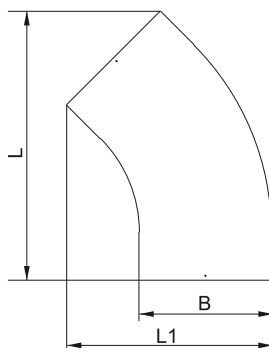
Рисунок 6 – Крышка поворота лестничного LESTA на 45 гр. R600 / Figure 6 – LESTA ladder cover 45 deg. turn R600 / 6-suret – LESTA satyly бүрлмасынүг қақпағу 45 гр. R600 / Рисунок 6 – Крышка повороту драбинного LESTA на 45 гр. R600
