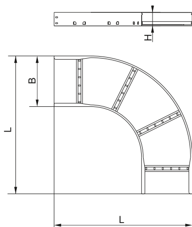
Рисунок 3 – Поворот лестничный LESTA на 90 гр. R300 / Figure 3 – LESTA ladder 90 deg. turn R300 / 3-suret – LESTA satyly бүрлмасы 90 гр. R300 / Рисунок 3 – Поворот драбинный LESTA на 90 гр. R300
