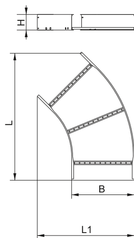
Рисунок 5 – Поворот лестничный LESTA на 45 гр. R600 / Figure 5 – LESTA ladder 45 deg. turn R600 / 5-suret – LESTA satyly бүрлмасы 45 гр. R600 / Рисунок 5 – Поворот драбинный LESTA на 45 гр. R600
