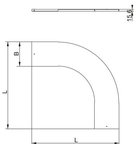
Рисунок 4 – Крышка поворота лестничного LESTA на 90 гр. R300 / Figure 4 – LESTA ladder cover 90 deg. turn R300 / 4-suret – LESTA satyly бүрлмасынүг қақпағу 90 гр. R300 / Рисунок 4 – Крышка повороту драбинного LESTA на 90 гр. R300
