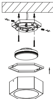
Рисунок 5 – Схема монтажа светильников типа 5204, 5304
