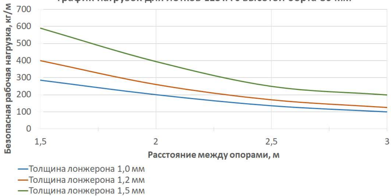
График нагрузок для лотков LESTA с высотой борта 80 мм
