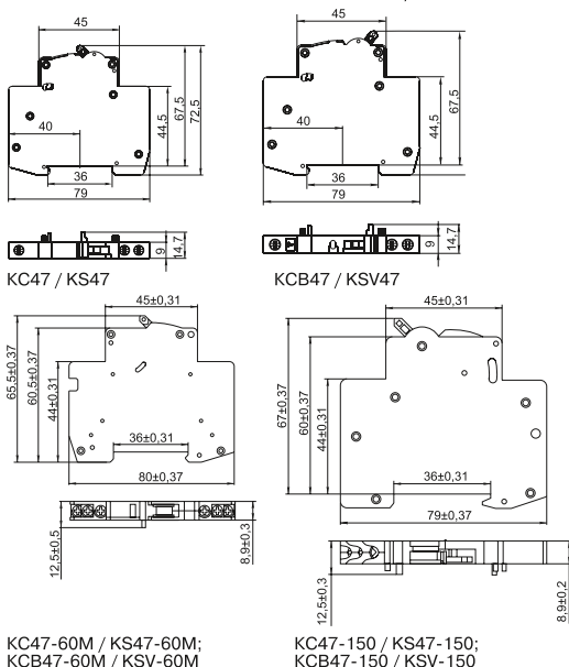
Рисунок 1 – Габаритные и установочные размеры устройств / Picture 1 – Overall and installation dimensions of devices
