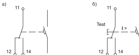
Рисунок 2 – Электрические схемы а) КС; б) КСВ / Picture 2 – Electric diagram a) KS; б) KSV
