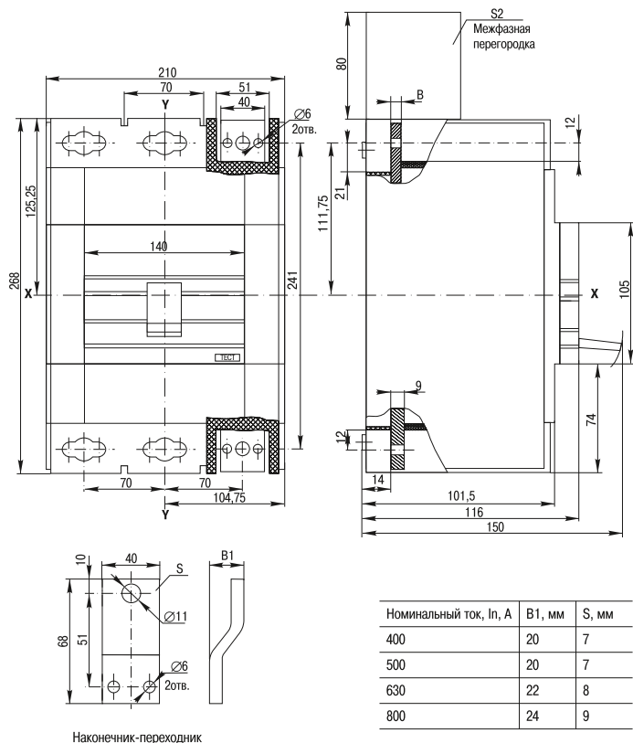
Рисунок 9 – Габаритные и установочные размеры выключателя BA88-40
